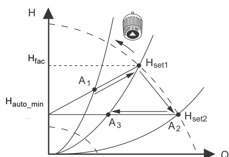
Fig. 50 AUTO ADAPT
