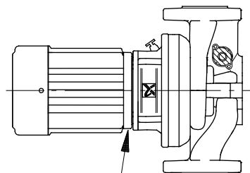
Fig. 136 Drain hole
