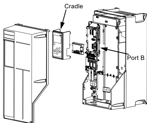
Fig. 172 Enclosures B2, C1
